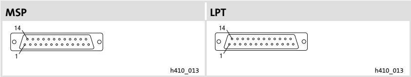
Abb. 2-1 DB25 Buchse
