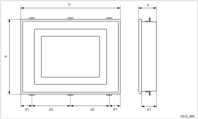
Fig.2-2 Encombrements
