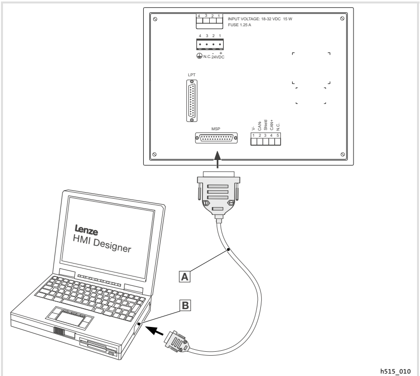
Fig.5-1 Relier l'unité de commande et le PC
