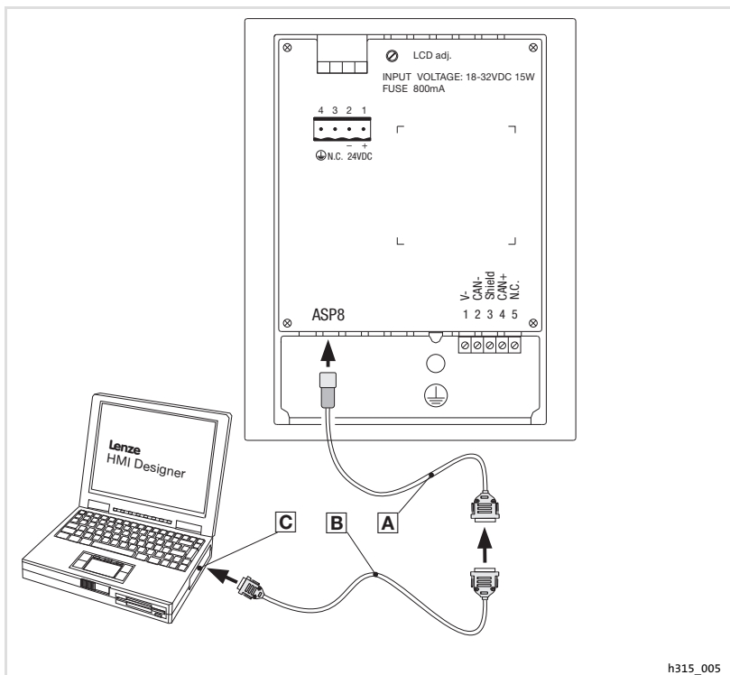
Fig.5-1 Etablissement de la liaison entre l'unité de commande au PC
