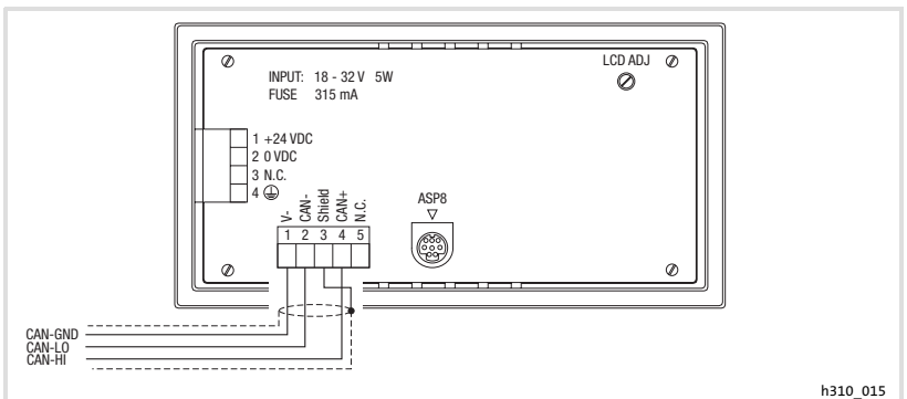
Abb. 4-3 Anschluss Systembus (CAN)
